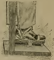
FIG. 24.—FOOT DYNAMOMETER.
